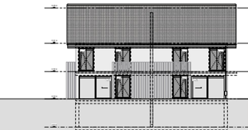
Südfassade
