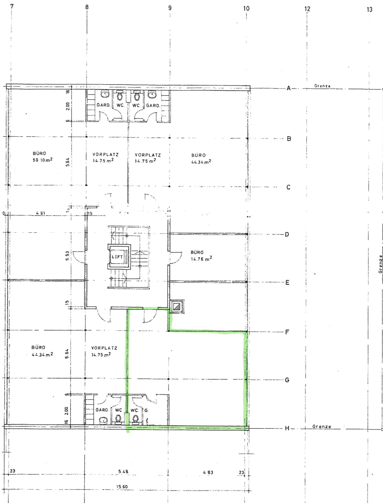
1. & 2. OBERGESCHOSS
