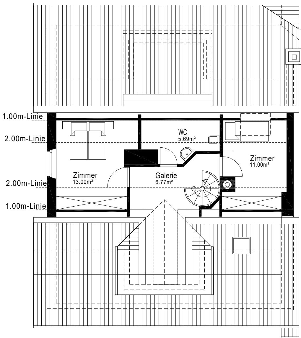
2.Dachgeschoss
